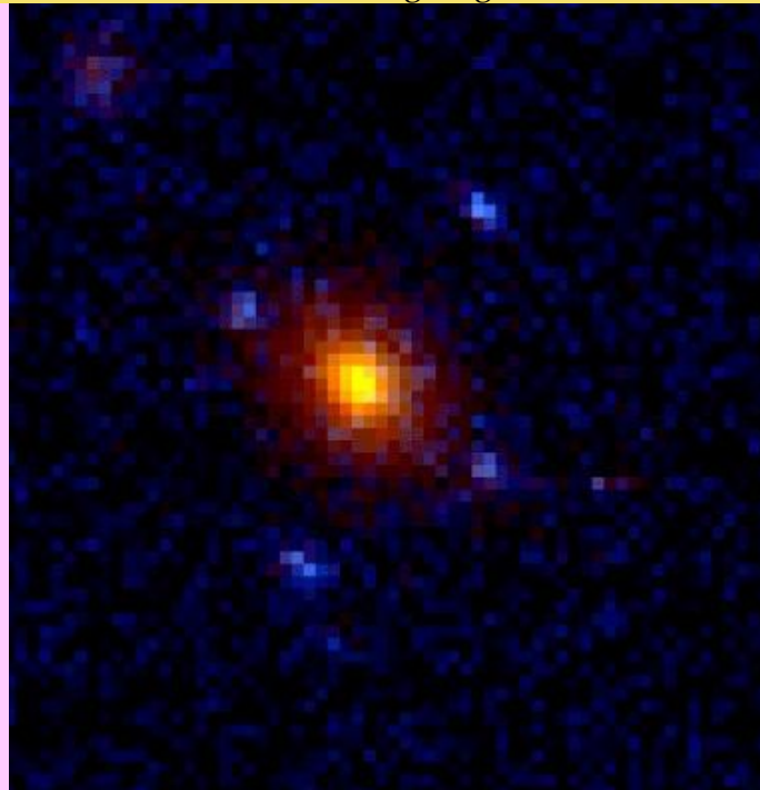
Foto einer "Gravitationslinse", die vielfache Bilder eines zentralen Objekts sichtbar macht.
